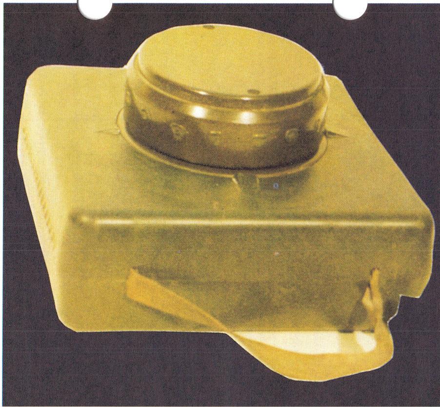
PRB M3 ANTITANK MINE
