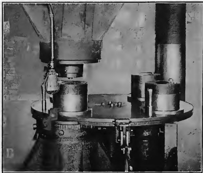
FIG. 5. INDENTING PRESS
