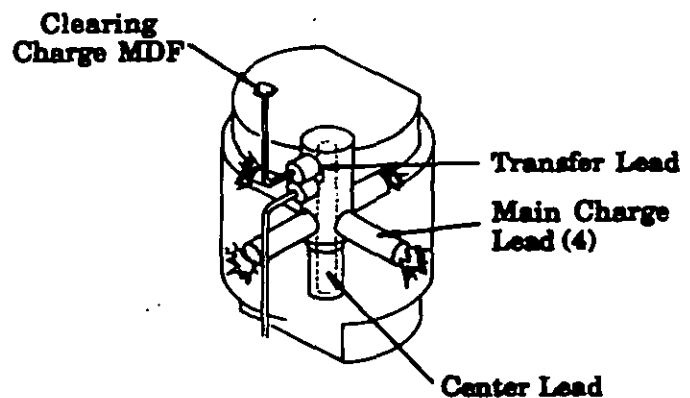
(D) Initiation of Explosive Train
