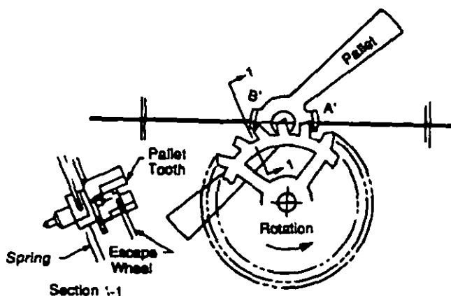
(D) Pallet at Equilibrium
