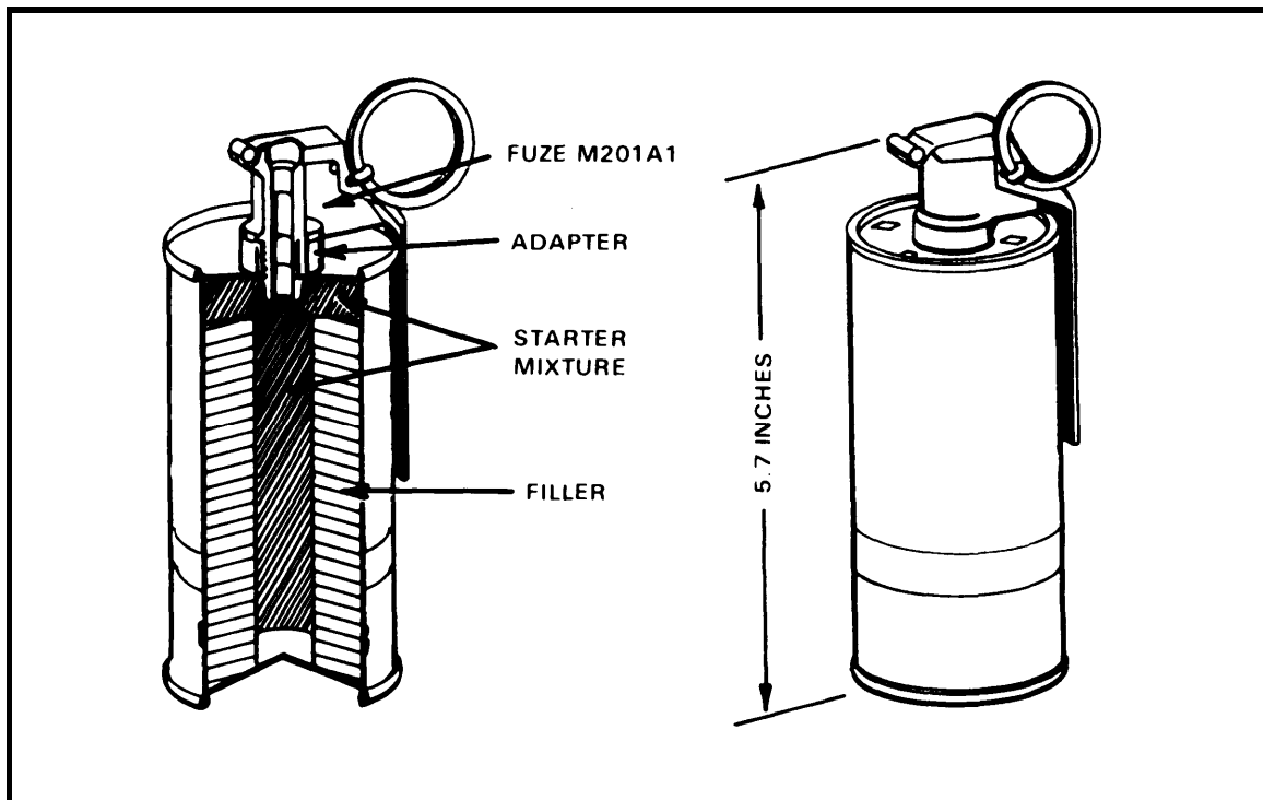
Figure D-6. ABC-M7A2 hand grenade.
