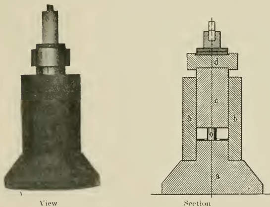
FIG. 103. Brisance Meter
